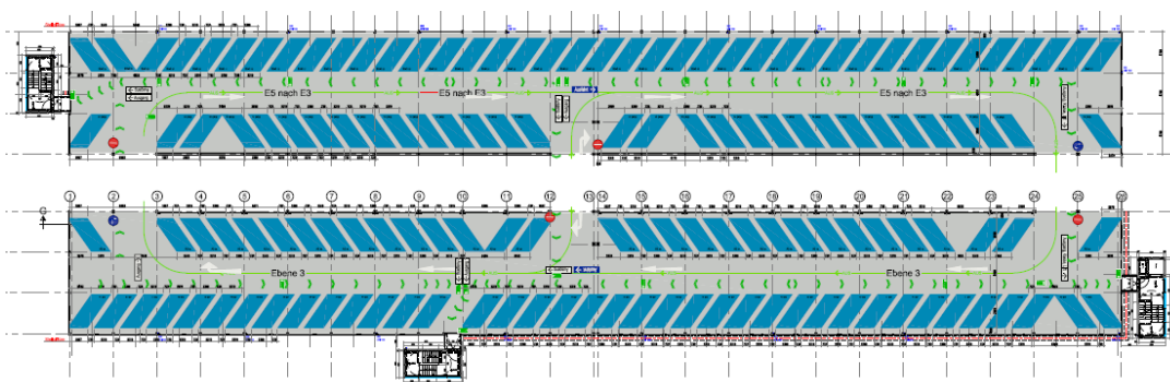
Grundriss Regelgeschoss
