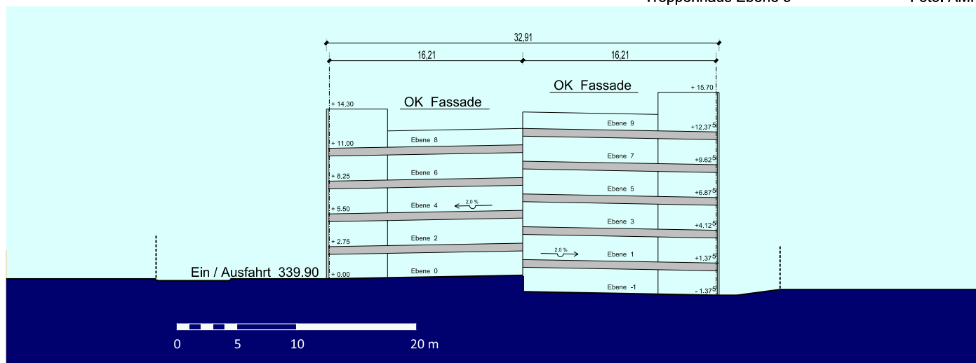
Systemschnitt
