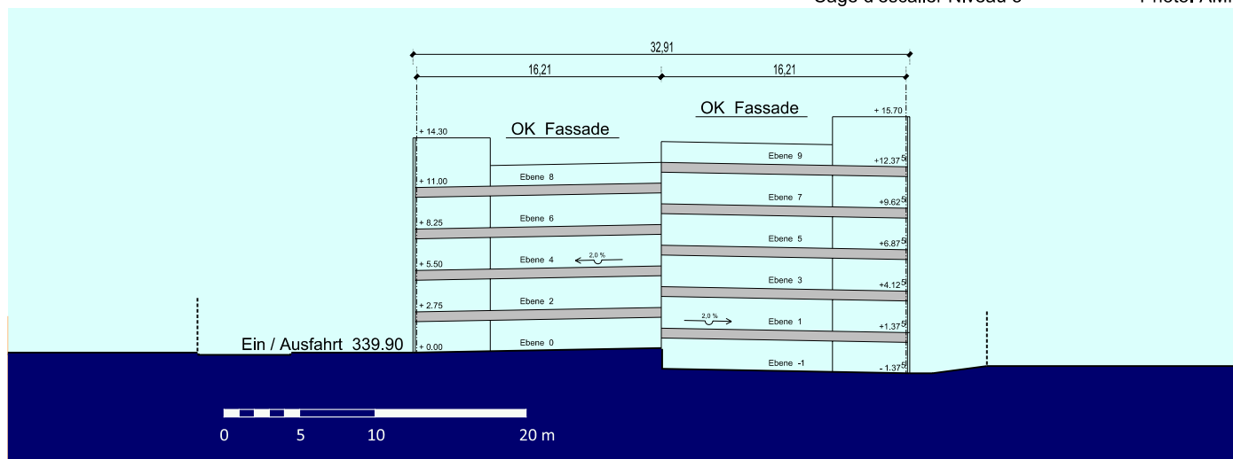
Coupe Système
